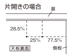
ラッチ取り付け下穴位置
